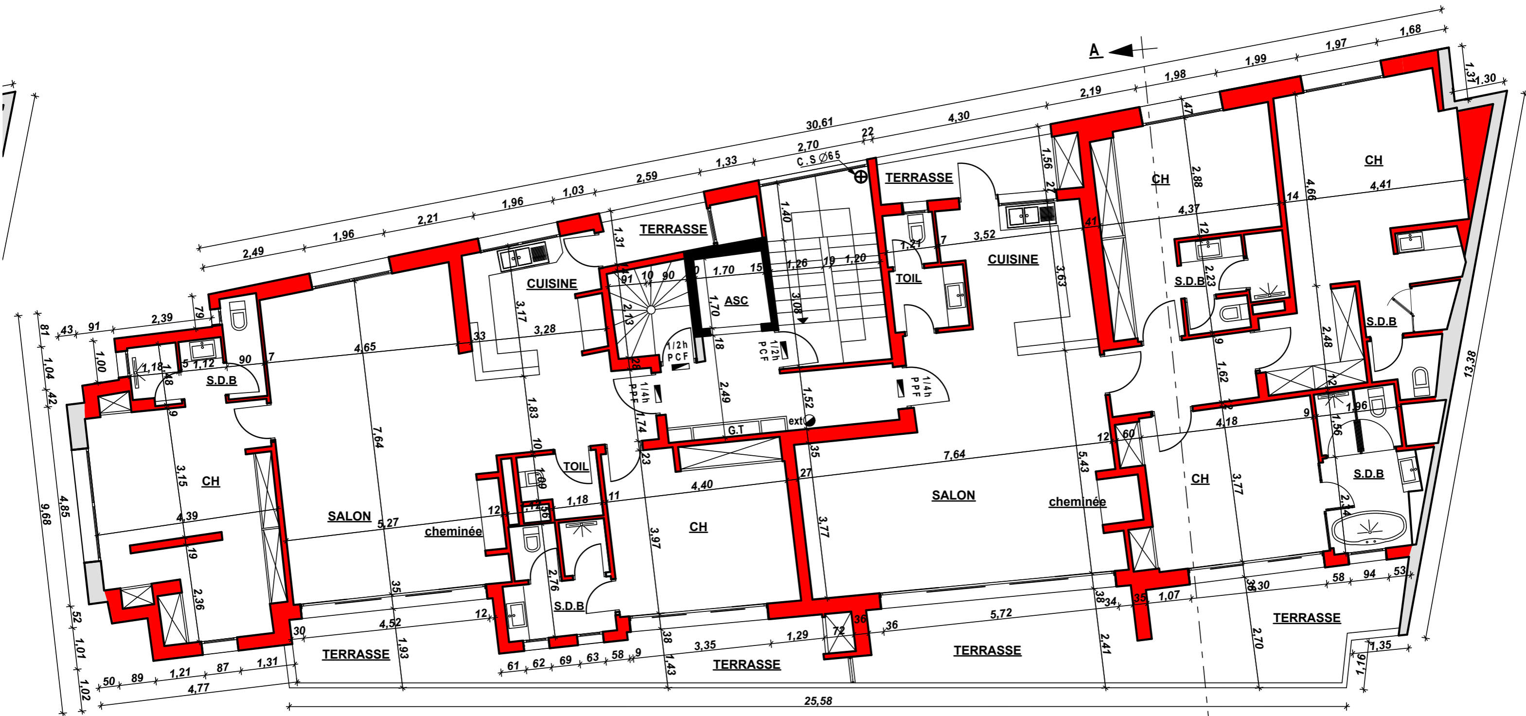
2è - 3è - 4è - 5è ETAGE MODIFIE
